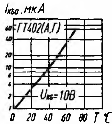
Зависимость обратного тока коллектора от температуры
